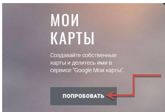
Рис. 2. Скриншот – инструкция
