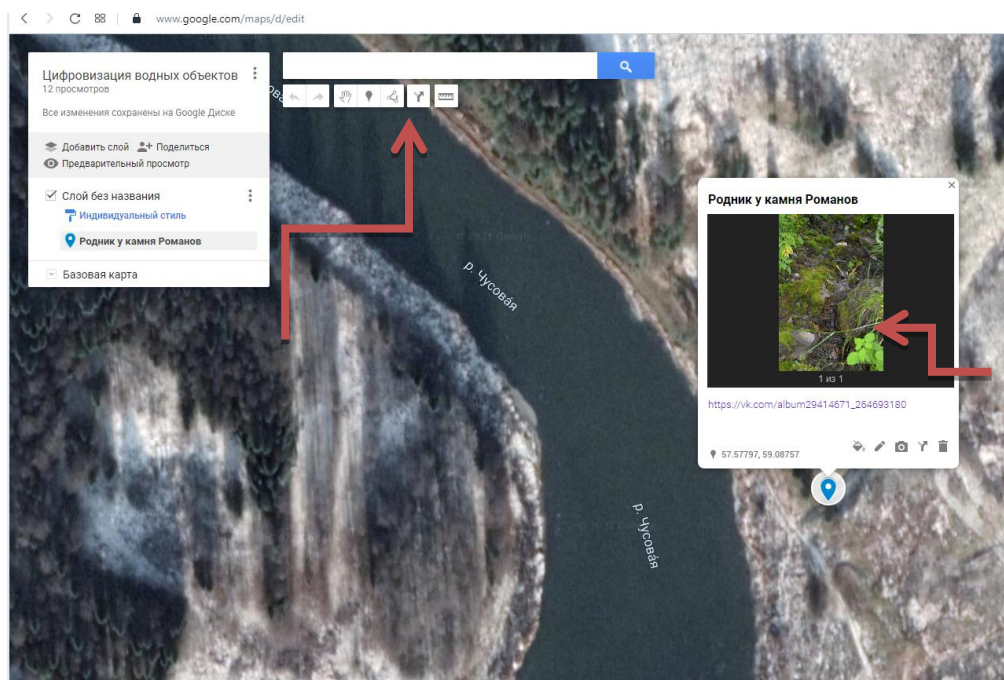
Рис. 4. Скриншот программы
